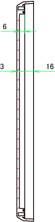
C-C ( 1 : 2.5 )
